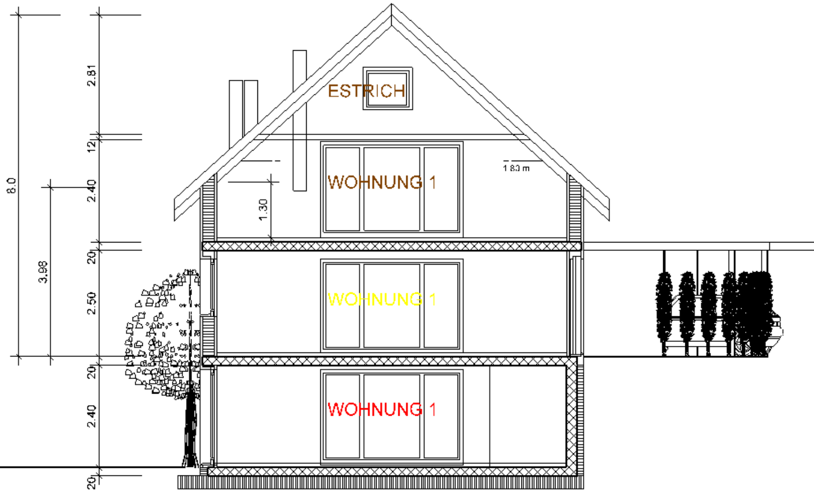
QUERSCHNITT MST. 1:100
